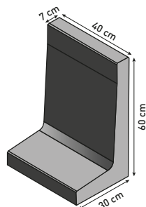
Mur en L 60 cm
