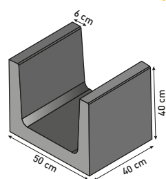
Mur en U 40 cm
