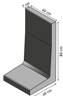
Mur en L 80 cm
