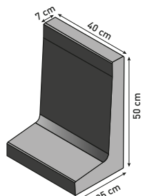
Mur en L 50 cm
