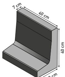
Mur en L 40 cm
